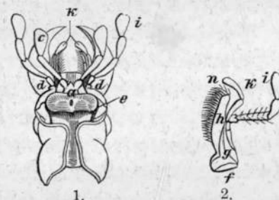
Рис. 5. Ротовые органы жуковъ. a — подбородокъ; c — губный щупалецъ; d — верхняя челюсть; e — нижняя челюсть, состоящая изъ слѣдующихъ частей: f — основной членикъ; g — стебелекъ; h и k — обѣ жевательныя пластинки; i — челюстное щупальце. — 1. Голова Procrustes coriaceus снизу. 2. Правая половинка нижней челюсти у Cicindela campestris .
