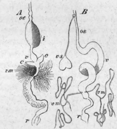
Рис. 8. — А. Пищевой каналъ полевого сверчка. В. Мухи. oe — пищеводъ; i — зобовидное расширение; v — желудокъ; c — его придатки; r — прямая кишка; vm — Мальпигіевы сосуды; vs — сосущій желудокъ.
