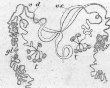
Рис. 12. — Мужскіе половые органы хруща ( Melolontha vulgaris ). tt — сѣмянники; vd — сѣменные протоки; vs — расширенный отдѣлъ ихъ; gl — извитыя придаточныя железы.
