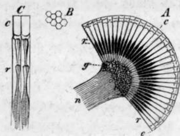
Рис. 4. — А. Схематическое изображеніе поперечнаго разрѣза сложнаго глаза членистоногихъ. n — зрительный нервъ; g — его узловое утолщеніе; r — кристаллики, начинающіеся изъ узла; c — граненая роговая оболочка, образовавшаяся изъ наружнаго покрова. Каждая грань вогнута внутрь и представляетъ свѣтопреломляющій органъ (хрусталикъ). В. Нѣсколько граней роговой оболочки съ поверхности. С. Кристаллики изъ глаза Procrustes coriaceus . r — палочки; c — роговая оболочка.
