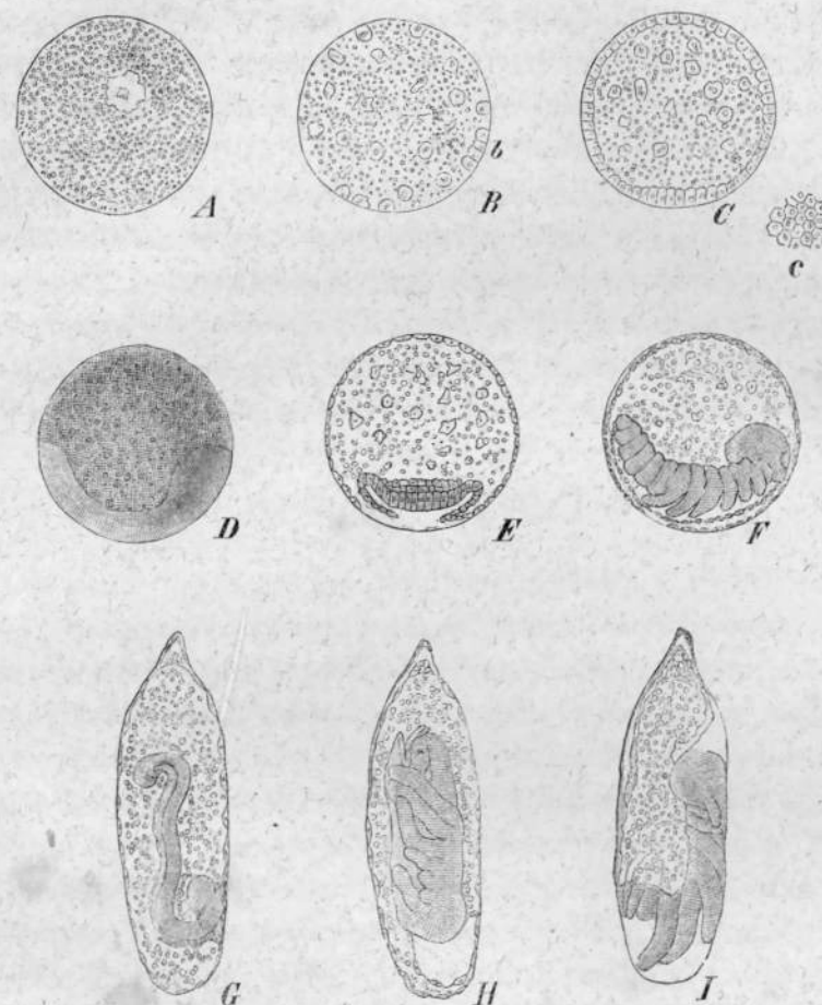
Рис. 14. — Отдѣльные моменты въ зародышномъ развитіи наѣжкомыхъ. (Объясненіе въ текстѣ).
