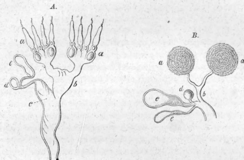
Рис. 10. — А. Женскіе половые органы у жука Platysoma frontale . aa — яйцевыя трубки; b — непарный яйцеводъ; c — совокупительный мѣшечекъ ( bursa copulatrix ); d — сѣмепріемникъ ( receptaculum seminis ); e — придаточная железа. — В. Женскіе половые органы у жука Meloe proscarabaeus .
