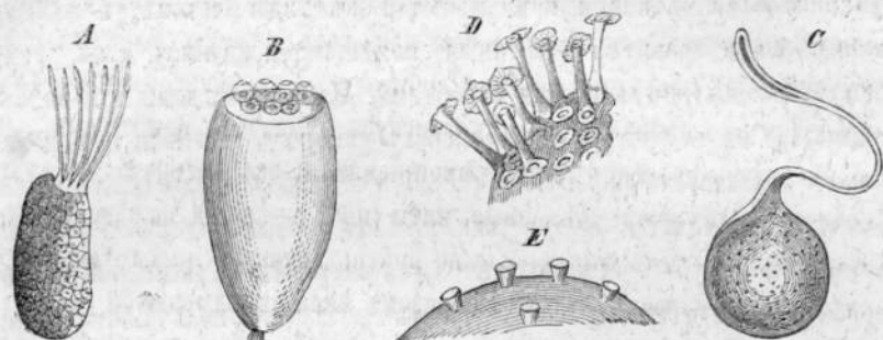
Рис. 13. — Аппаратъ Mikropyle у яицъ разныхъ насѣкомыхъ. — А. Водяного клопа Nera cinerea (яйцо снято въ профили). В. Головной вши ( Pediculus capitis ). С. Оканчивающееся глухимъ рукавомъ яйцо орѣхотворки Cynips quercus . D. Кусокъ скорлупы ( chorion ) яйца кузнечика Locusta viridissima . E. Верхній полюсъ яйца (съ микропилями) клопа Pyrrhocoris apterus .
