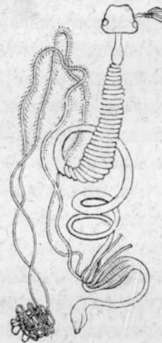
Рис. 7. — Кишечный каналъ хруща ( Melolontha vulgaris ) съ частію перистыми Мальпигіевыми сосудами (съ правой стороны отрѣзанными).
