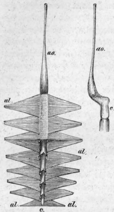
Рис. 9. — А. Спинной сосудъ хруща ( Melolontha vulgaris ). c — раздѣленное на камеры сердце; ao — аорта, идущая въ грудь; al — такъ назыв. крыловидныя мышцы, прикрѣпляющіяся по бокамъ сердца. — В. Аорта, съ первою камерою сердца, съ боку.
