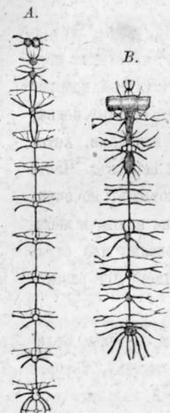
Рис. 3. Брюшная нервная цѣпь бражника Sphinx ligustri . А — гусеницы; В — бабочки.
