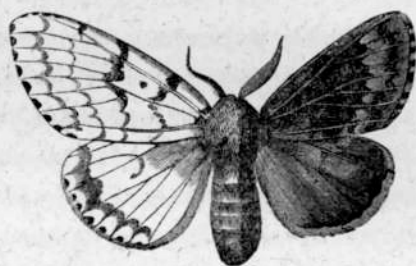
Рис. 15. — Боковой гермафродитъ непарнаго шелкопряда ( Ocneria dispar ).
